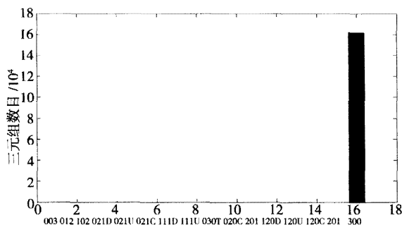
图 6 群体观点选择状态两极化后的三元组结构关系分布 (其中编码 300 对应三元组结构中的结构平衡关系)
