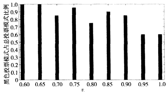
图 7 v_s 对群体观点极化的影响(固定 \varepsilon = 0.01, \lambda = 0.01 )
